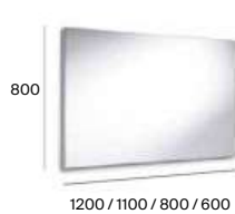
1200 / 1100 / 800 / 600
