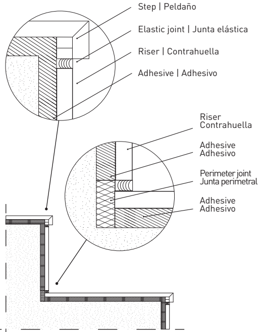
Detail of steps on a staircase / Detalle de peldaños en escalera (UNE 138002:2017)
