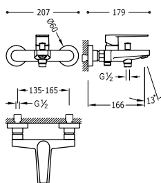
Grifo monomando mural para bañera y ducha Ducha de mano anticalcárea. Soporte orientable para ducha de mano. Flexo satinado.
