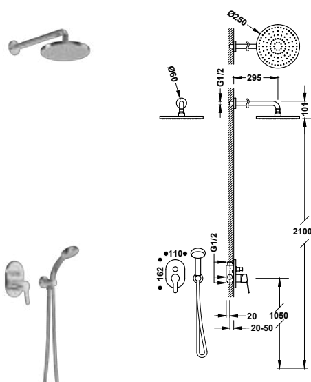
Kit de grifo monomando empotrado de 2 vías para ducha
