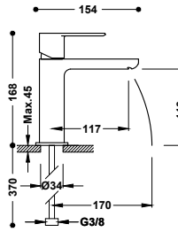
Grifo monomando para lavabo Caño cerrado con salida del agua en cascada. Latiguillos de alimentación flexibles G3/8. Se incluyen 2 llaves de regulación con filtro (ref: 9134525).
