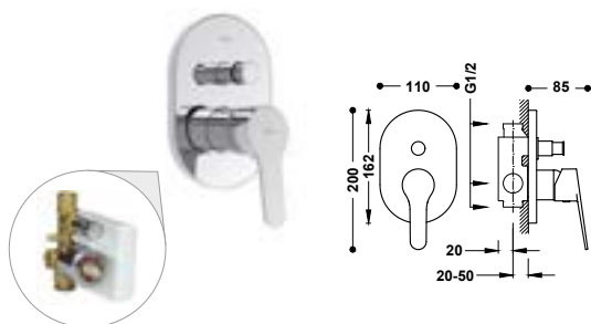
Grifo monomando empotrado de 2 vías para bañera y ducha Cuerpo empotrado incluido. Inversor de 2 vías.
