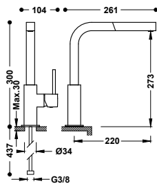
Grifo monomando con caño extraíble para cocina Con latiguillos de alimentación flexible G3/8.
