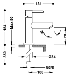
Grifo monomando para lavabo Latiguillos de alimentación flexibles G3/8.
