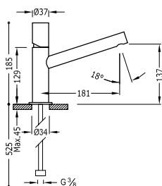
Grifo monomando para lavabo Caño largo. Latiguillos de alimentación flexibles G3/8.
