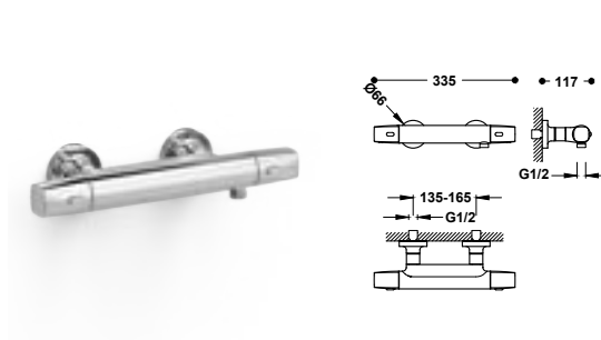
Grifo termostático mural Over-wall para ducha Sin complementos. Volante con bordes redondeados.
