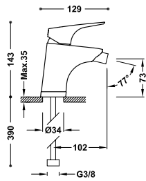
Grifo monomando para bidé Latiguillos de alimentación flexibles G3/8.
