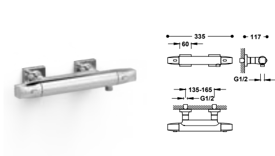
Grifo termostático mural Over-wall para ducha Sin complementos. Volante cuadrado-redondo.
