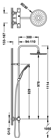
Conjunto de grifo termostático mural Over-wall de 2 vías para ducha
