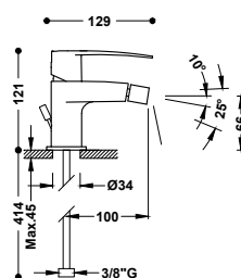
Grifo monomando para bidé Latiguillos de alimentación flexibles G3/8.
