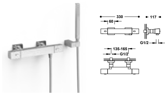
Grifo termostático mural Over-wall para ducha Ducha de mano anticalcárea de latón. Soporte orientable para ducha de mano. Flexo satinado. Volante cuadrado.
