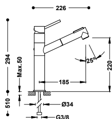
Grifo monomando con caño extraíble con 2 tipos de chorro para cocina Con latiguillos de alimentación flexibles G3/8.
