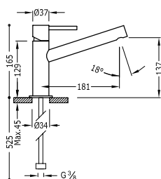
Grifo monomando para lavabo Caño largo. Latiguillos de alimentación flexibles G3/8.
