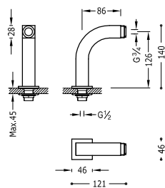
Tomas de agua acodadas de instalación a borde bañera para grifo de bañera
