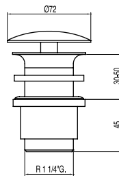
Válvula de desagüe siempre abierto para lavabo sin rebosadero
