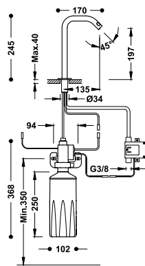
Grifo electrónico de 1 agua con dispensador de jabón automático para lavabo
