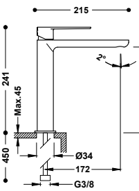
Grifo monomando alto para lavabo Latiguillos de alimentación flexibles G3/8.
