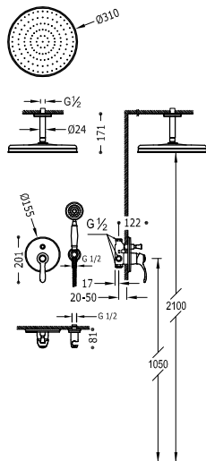
Kit de grifo monomando empotrado de 2 vías para ducha
