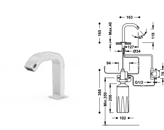
Grifo electrónico de 1 agua con dispensador de jabón automático para lavabo
