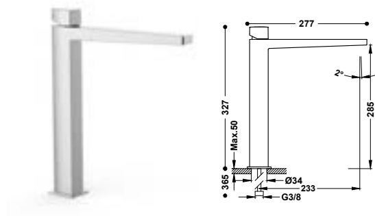
Grifo monomando XXL para lavabo Latiguillos de alimentación flexibles G3/8.
