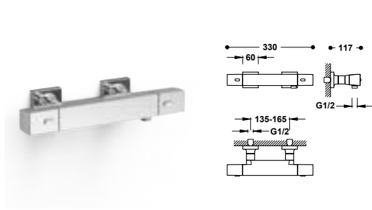
Grifo termostático mural Over-wall para ducha Sin complementos. Volante cuadrado.
