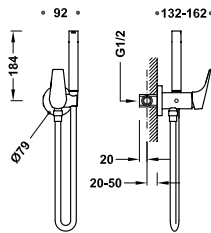
Grifo monomando empotrado con ducha para inodoro Con agua fría o caliente. Ducha de mano con racor limitador a 5 l/min. y sistema antigoteo. Soporte fijo para la ducha de mano instalable a derecha o izquierda. Flexo satinado.
