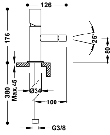
Grifo monomando para bidé Rótula orientable. Latiguillos de alimentación flexibles G3/8.
