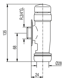
Grifo de descarga temporizado mural de 1 agua para urinario
