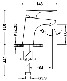
Grifo monomando ecoeficiente para lavabo Latiguillos de alimentación flexibles G3/8.
