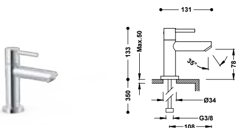
Grifo de 1 agua para lavabo Con latiguillo de alimentación flexible G3/8.
