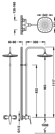
Conjunto de grifo monomando mural de 1 vía para ducha · Rociador de ducha orientable: 242x242 mm.
