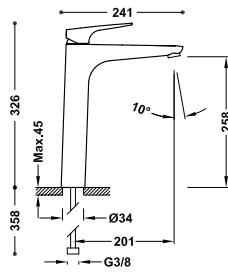
Grifo monomando XXL para lavabo Latiguillos de alimentación flexibles G3/8.
