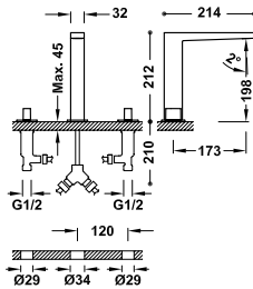
Grifo bimando de repisa para lavabo De instalación libre. Con volantes.
