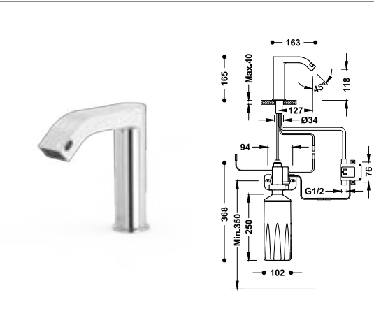
Grifo electrónico de 1 agua con dispensador de jabón automático para lavabo
