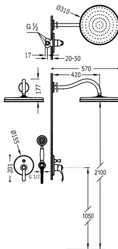
Kit de grifo monomando empotrado de 2 vías para ducha
