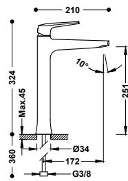
Grifo monomando XXL para lavabo Latiguillos de alimentación flexibles G3/8.
