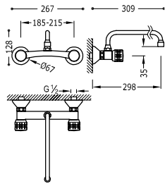
Grifo bimando mural para cocina Con caño superior. Excentricidad especial. Distancia a pared: 298 mm.
