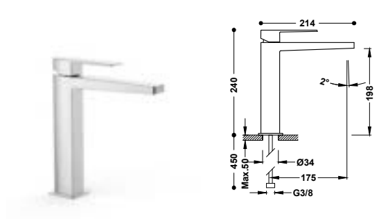
Grifo monomando alto para lavabo Latiguillos de alimentación flexibles G3/8.
