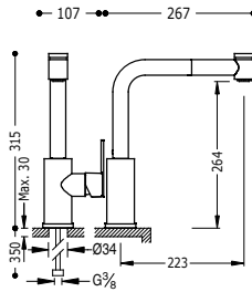
Grifo monomando con caño extraíble con 2 tipos de chorro para cocina Con latiguillos de alimentación flexible G3/8.
