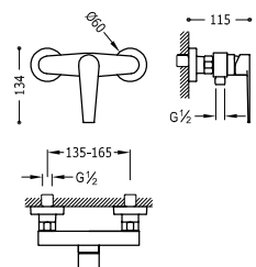
Grifo monomando mural para ducha Ducha de mano anticalcárea. Soporte orientable para ducha de mano. Flexo satinado.
