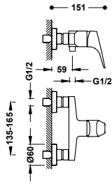
Grifo monomando mural para ducha Sin complementos.
