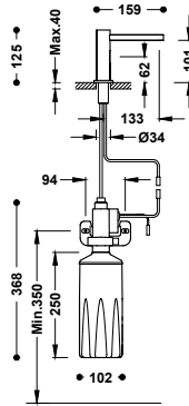
Dispensador electrónico de jabón para lavabo y cocina Accionado mediante sensor de infrarrojos. Capacidad del depósito de jabón: 1.600 ml.
