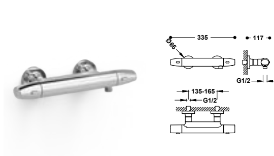
Grifo termostático mural Over-wall para ducha Sin complementos. Volante ovalado.
