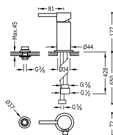
Grifo monomando para bidé con transferencia a duchita Con inversor para duchita. Latiguillos de alimentación flexibles G3/8.
