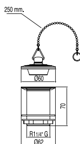
Válvula de desagüe con tapón y cadenilla para lavabo sin rebosadero Cadenilla de 250 mm.
