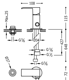
Grifo monomando para bidé con transferencia a ducha Latiguillos de alimentación flexibles G3/8.
