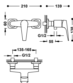
Grifo monomando mural para ducha Ducha de mano anticalcárea 120x120 mm. (3 tipos de chorro). Soporte orientable para ducha de mano. Flexo metálico.
