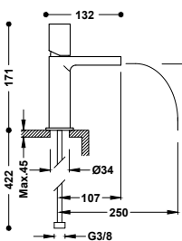
Grifo monomando para lavabo Caño abierto con salida del agua en cascada. Latiguillos de alimentación flexibles G3/8. Se incluyen 2 llaves de regulación con filtro (ref: 9134525).
