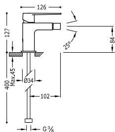
Grifo monomando para bidé Rótula orientable. Latiguillos de alimentación flexibles G3/8.
