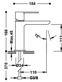
Grifo monomando para lavabo Latiguillos de alimentación flexibles G3/8.
