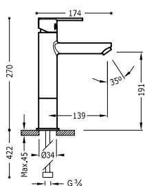
Grifo monomando alto para lavabo Con aireador de fácil limpieza. Latiguillos de alimentación flexibles G3/8.
