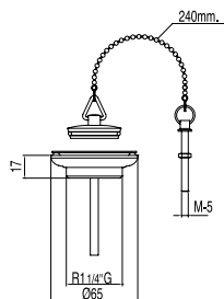
Cazoleta plana de desagüe con kit de enganche de cadena y tapón para lavabo, bidé y fregadero Cadenilla de 240 mm.
