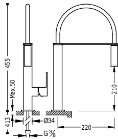
Grifo monomando con caño flexible para cocina Con latiguillos de alimentación flexible G3/8.
