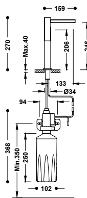
Dispensador electrónico alto de jabón para lavabo y cocina Accionado mediante sensor de infrarrojos. Capacidad del depósito de jabón: 1.600 ml.
