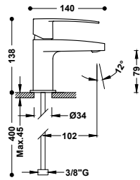
Grifo monomando para lavabo Latiguillos de alimentación flexibles G3/8.
