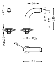
Tomas de agua acodadas de instalación a borde bañera para grifo de bañera 2 unidades con silenciador.
