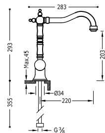
Grifo monomando para cocina Con latiguillos de alimentación flexibles G3/8.
