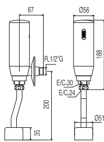
Grifo de descarga electrónico mural de 1 agua para urinario Accionado mediante sensor de infrarrojos. Con dos tubos adaptables a urinario.
