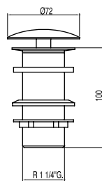
Válvula de desagüe siempre abierto para lavabo sin rebosadero
