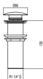
Válvula de desagüe Click-Clack para lavabo sin rebosadero Sin rebosadero. Función Click-Clack. Tapón: Ø 66 mm.
