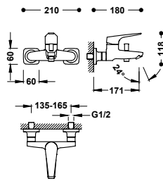
Grifo monomando mural para bañera y ducha Ducha de mano anticalcárea 120x120 mm. (3 tipos de chorro). Soporte orientable para ducha de mano. Flexo metálico.
