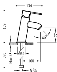
Grifo monomando inclinado para lavabo Con aireador de fácil limpieza. Latiguillos de alimentación flexibles G3/8.
