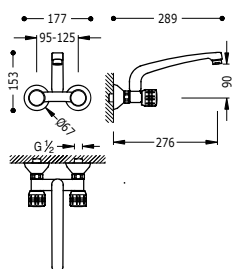
Grifo bimando mural para cocina Con caño superior. Excentricidad especial. Distancia a pared: 276 mm.
