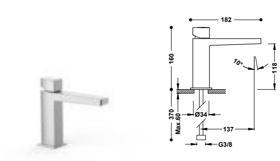
Grifo monomando para lavabo Latiguillos de alimentación flexibles G3/8.
