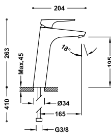
Grifo monomando alto para lavabo con Tres-Duo Latiguillos de alimentación flexibles G3/8.
