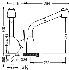
Grifo monomando con caño extraíble con 2 tipos de chorro para cocina Con latiguillos de alimentación flexibles G3/8.
