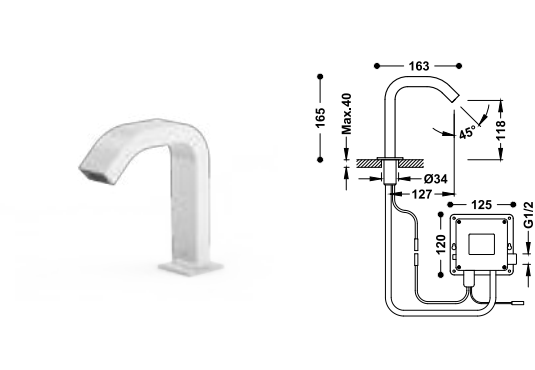
Grifo electrónico de 1 agua para lavabo Accionado mediante sensor de infrarrojos.
