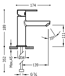
Grifo monomando para lavabo Con aireador de fácil limpieza. Latiguillos de alimentación flexibles G3/8.
